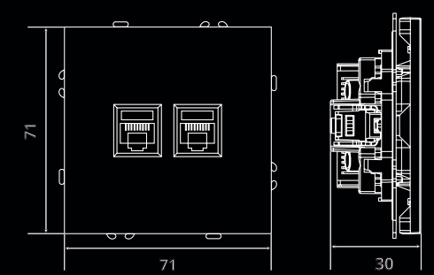
Розетка компьютерная 2-местная RJ-45 (механизм)
