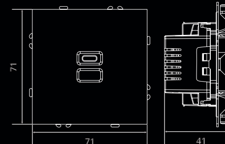
Розетка 2-местная USB + Type C (механизм), 20Вт
