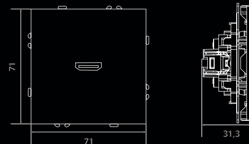
Розетка 1-местная HDMI 2.0 Type A (механизм)
