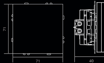
Переключатель 1-клавишный (механизм), 10А
