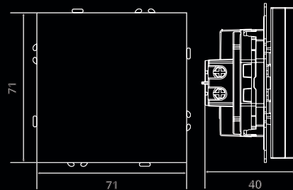
Переключатель перекрестный 1-клавишный (механизм), 10А
