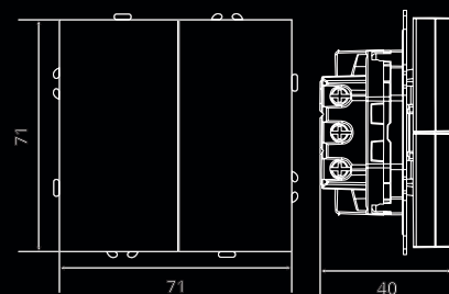
Выключатель 2-клавишный с индикатором (механизм), 10А
