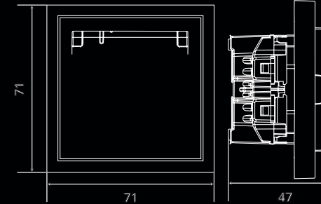
Розетка 1-местная с крышкой с защитной шторкой с/з (механизм), 16А, IP42
