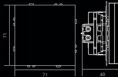
Выключатель 1-клавишный (механизм), 10А
