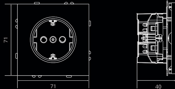
Розетка 1-местная с защитной шторкой с/з (механизм), 16А, IP20
