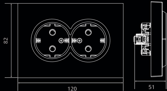
Розетка 2-местная с защитной шторкой с/з, 16А, IP20
