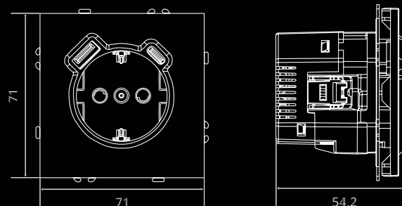
Розетка 1-местная с/ш, с/з (механизм), 16А + USB + Type C
