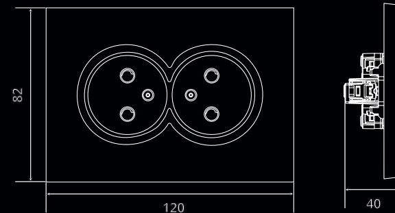
Розетка 2-местная с защитной шторкой б/з, 16А, IP20
