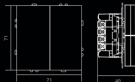
Переключатель перекрестный 2-клавишный (механизм), 10А
