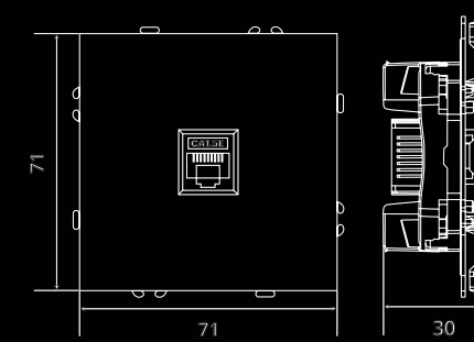
Розетка компьютерная 1-местная RJ-45 (механизм)
