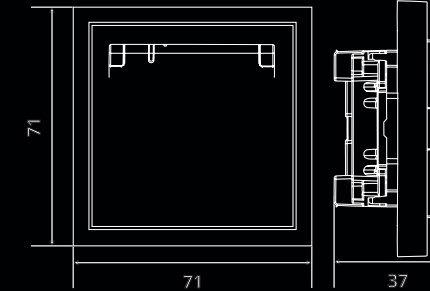
Розетка 1-местная с крышкой с защитной шторкой б/з (механизм), 16А, IP42
