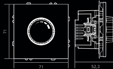
Выключатель диммирующий (механизм), 2А, 500Вт
