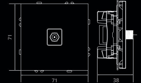
Розетка телевизионная 1-местная 75 Ом, 5-862МГц (механизм)
