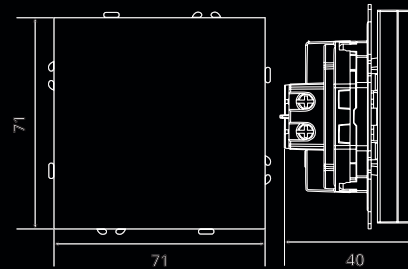
Выключатель 1-клавишный с индикатором (механизм), 10А
