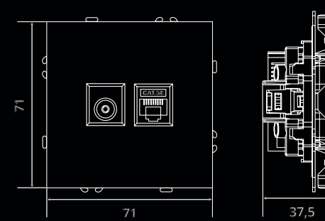
Розетка TV + компьютерная RJ-45 (механизм)
