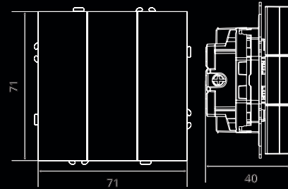
Выключатель 3-клавишный (механизм), 10А
