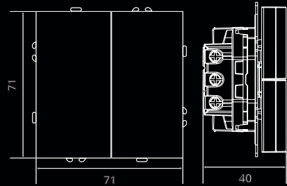
Выключатель/Переключатель 2-клавишный (механизм), 10А
