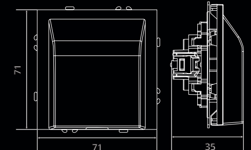
Кабельный вывод (механизм)
