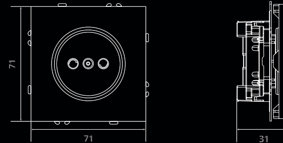
Розетка 1-местная с защитной шторкой б/з (механизм), 16А, IP20
